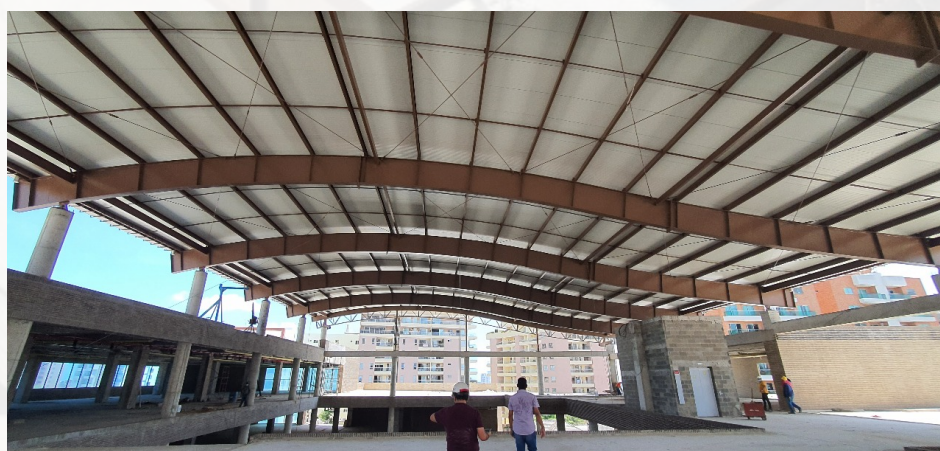
Cubierta centro comercial Le Meridien Barranquilla
